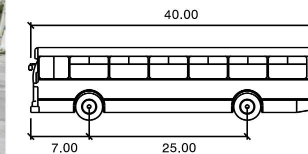
CITY-BUS Width : 8.50
